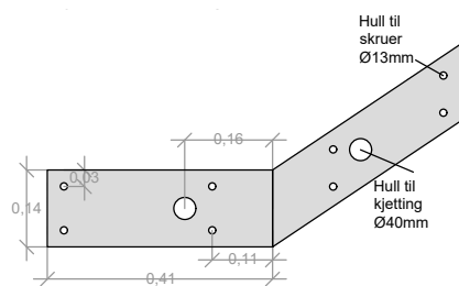
Hjørnebeslag
