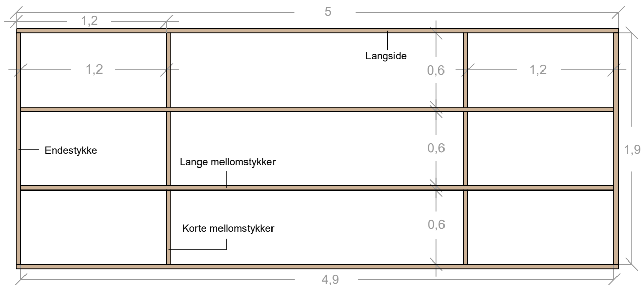
Skisse over rammen til badeflåten
