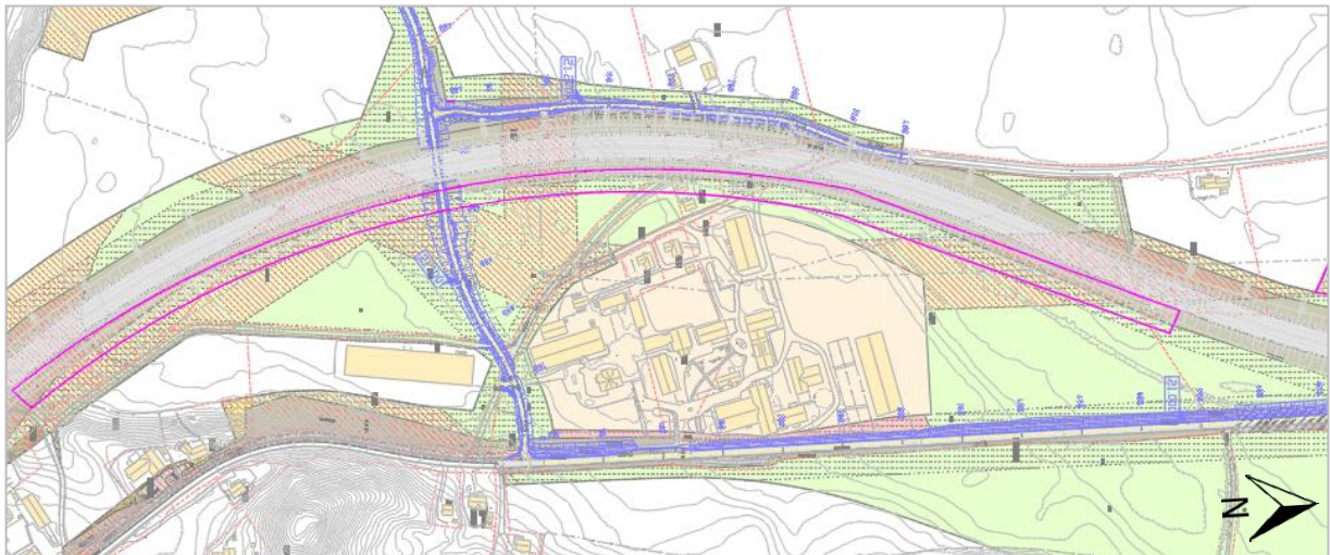
Figur 7: Utsnitt av gjeldende reguleringsplan og justert veggeometri rundt Øya
