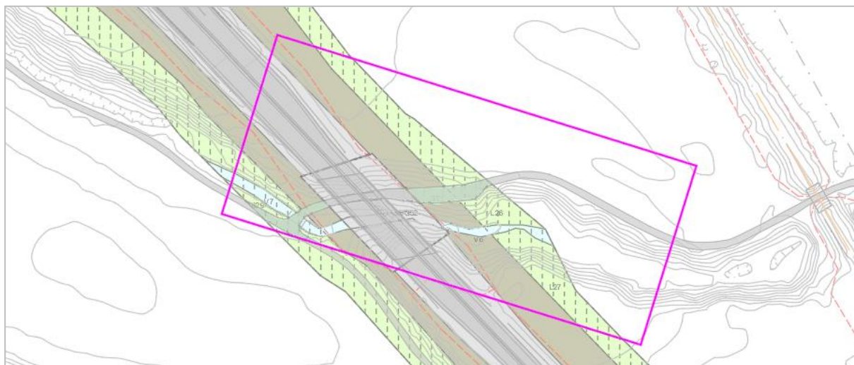
Figur 21: Utsnitt av gjeldende reguleringsplan og justert veggeometri rundt Lodbekken
