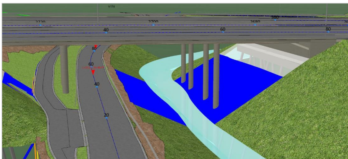
Figur 18: Kvålsbekken i permanent situasjon, Bennavegen til venstre (Kilde: Novapoint-modell)
