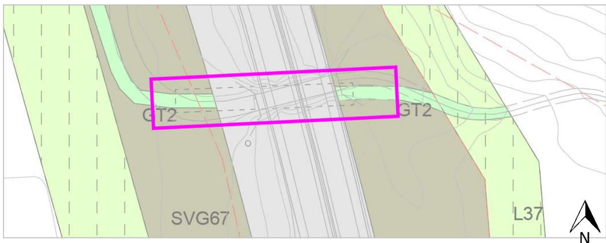
Figur 27: Utsnitt av gjeldende reguleringsplan og justert veggeometri rundt kulvert profil 8300
