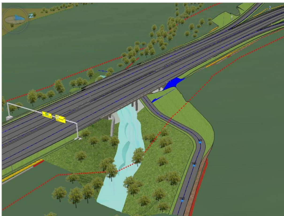
Figur 22: Viser Lodbekken, bru og driftsveg med skråningsutslag (Kilde: Novapoint-modell)
