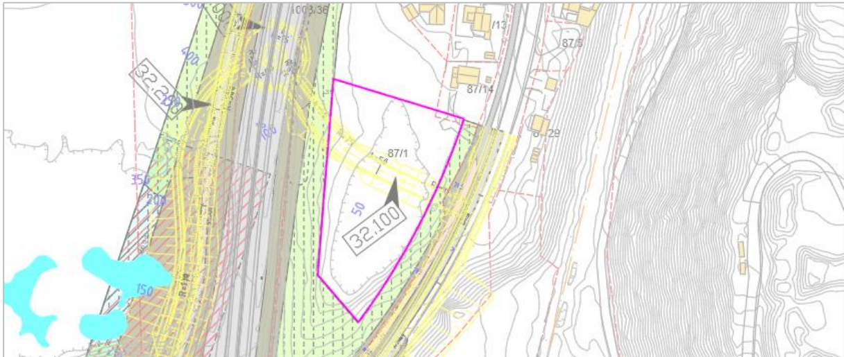
Figur 14: Utsnitt av gjeldende reguleringsplan og justert veggeometri rundt gnr./bnr. 87/1
