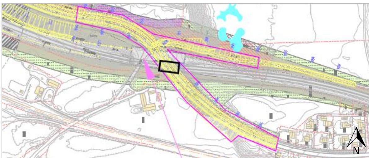
Figur 23: Utsnitt av gjeldende reguleringsplan og justert veggeometri rundt Hofstadtunnelen
