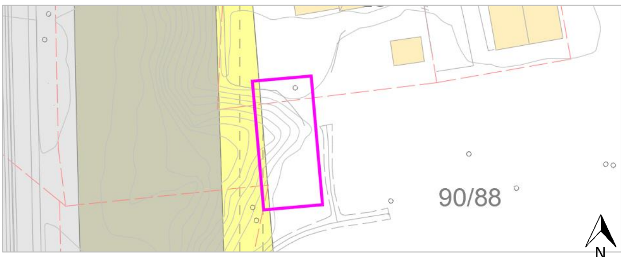
Figur 15: Utsnitt av gjeldende reguleringsplan og justert veggeometri rundt gnr./bnr. 90/25 og 88
