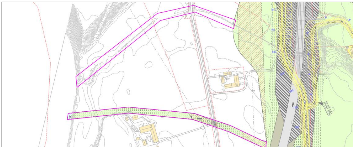
Figur 25: Utsnitt av gjeldende reguleringsplan og justert veggeometri rundt overvanns-/drenskanal Øya
