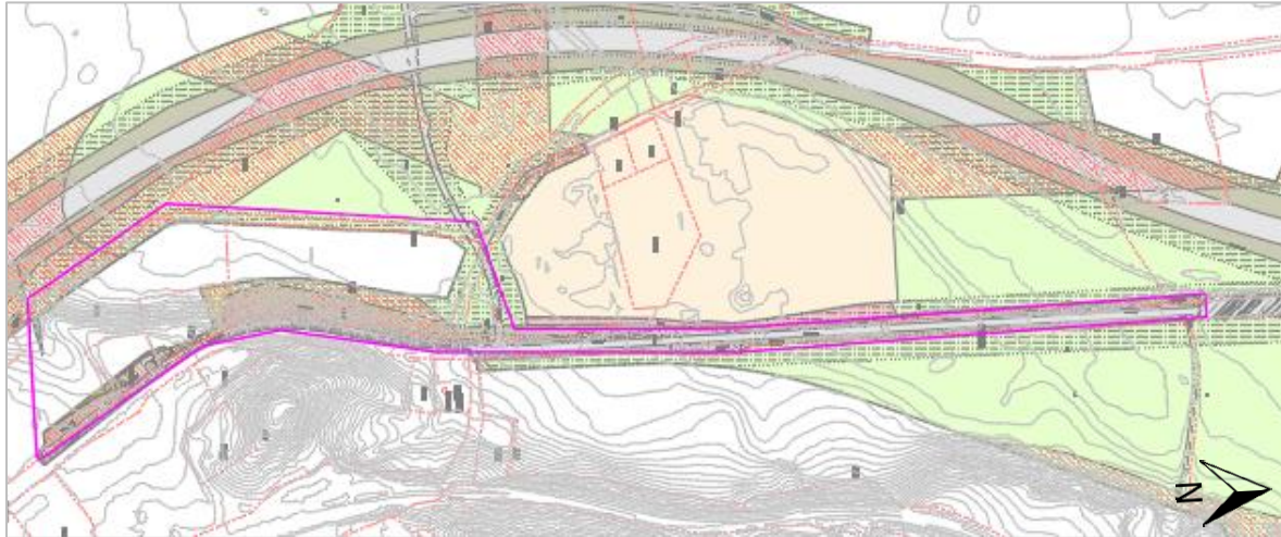
Figur 12: Utsnitt av gjeldende reguleringsplan og justert veggeometri rundt GS-veger på Øya
