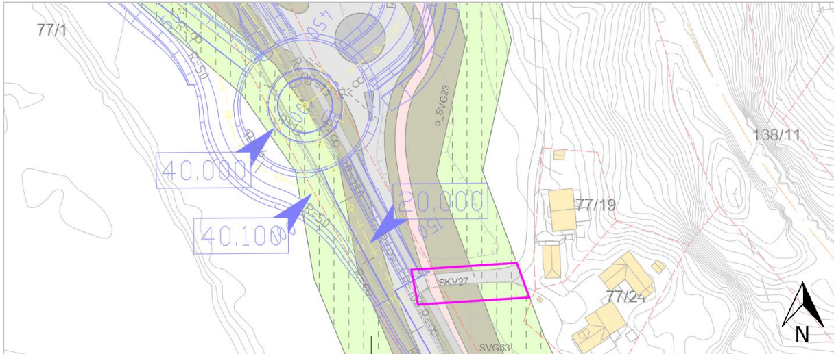
Figur 19: Utsnitt av gjeldende reguleringsplan og justert veggeometri rundt adkomst til gnr./bnr. 77/19 og 24
