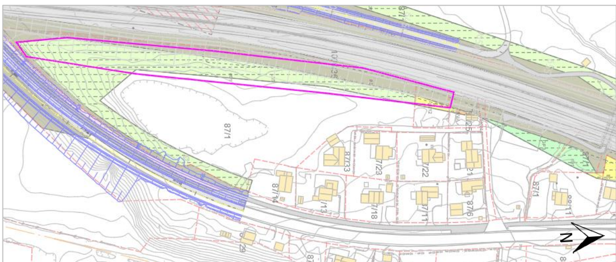
Figur 8: Utsnitt av gjeldende reguleringsplan og justert veggeometri rundt Søberg
