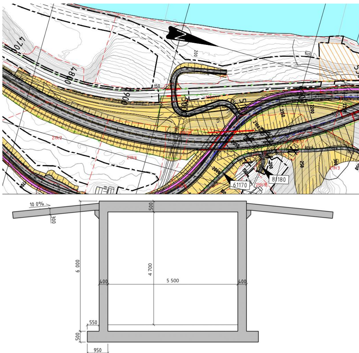
Figur 7-5 Tverrsnittet viser planlagt dimensjon for undergang under jernbane ved Røskaft.
