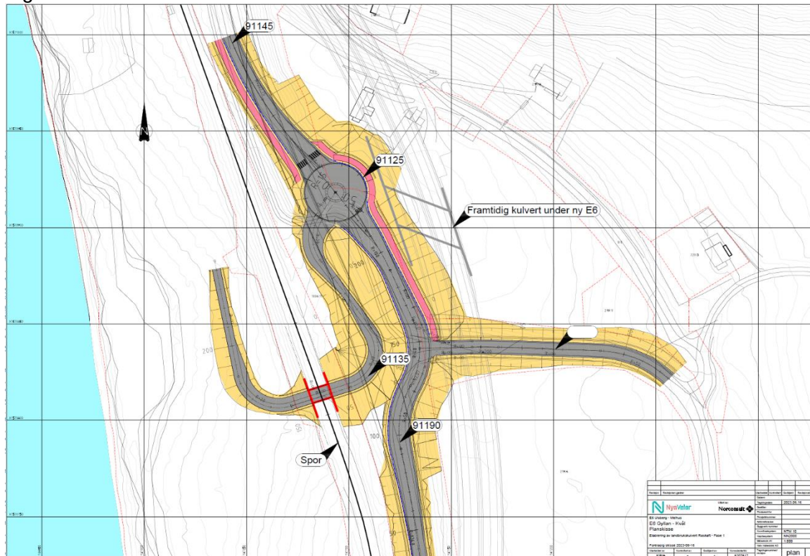
Figur 7-3 Skisse av mulig løsning for kobling mellom dagens E6 og ny jernbaneundergang som kan etableres i byggefasen.
