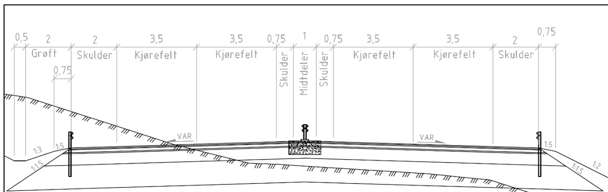
Figur 4-2: H3-profil med veibredde 20,5 m [74].
